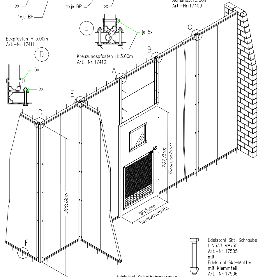
GFK U-Pfosten L: 3.31m Art.-Nr.: 17657
