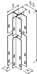
Edelstahl Kreuzungspfosten H: 3.00m Art.-Nr.: 17410
