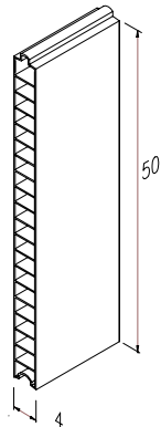
Brettprofil BP 500x40 max. 7.00m Lang
