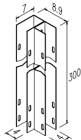
Edelstahl Eckpfosten H: 3.00m Art.-Nr.: 17411
