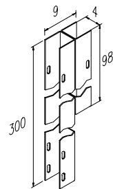
Edelstahl Türpfostenprofil mit Sturzaufnahme H: 3.00m Art.-Nr.: 17408
